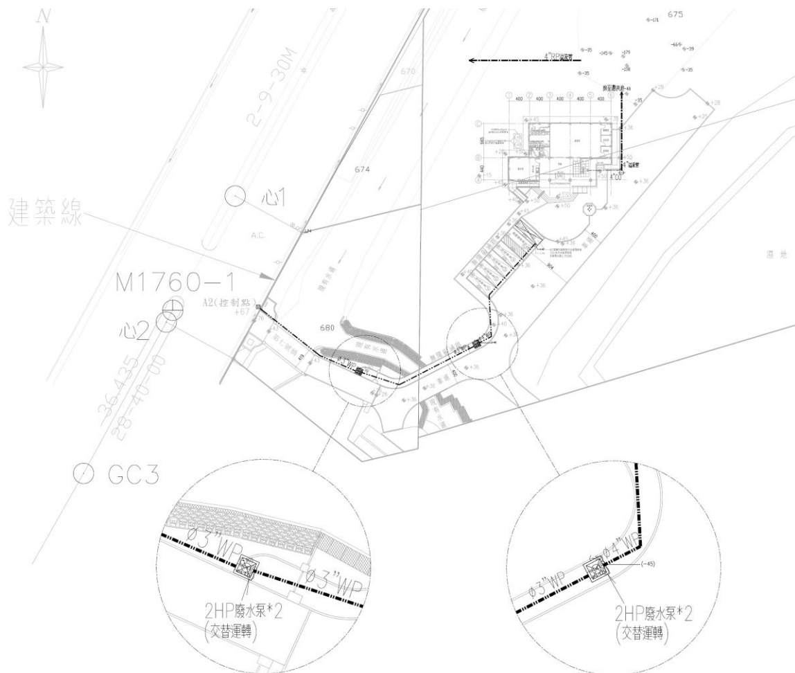
圖 8-9、全區雨污水分流配置平面圖(林愷歆建築師事務所提供)
