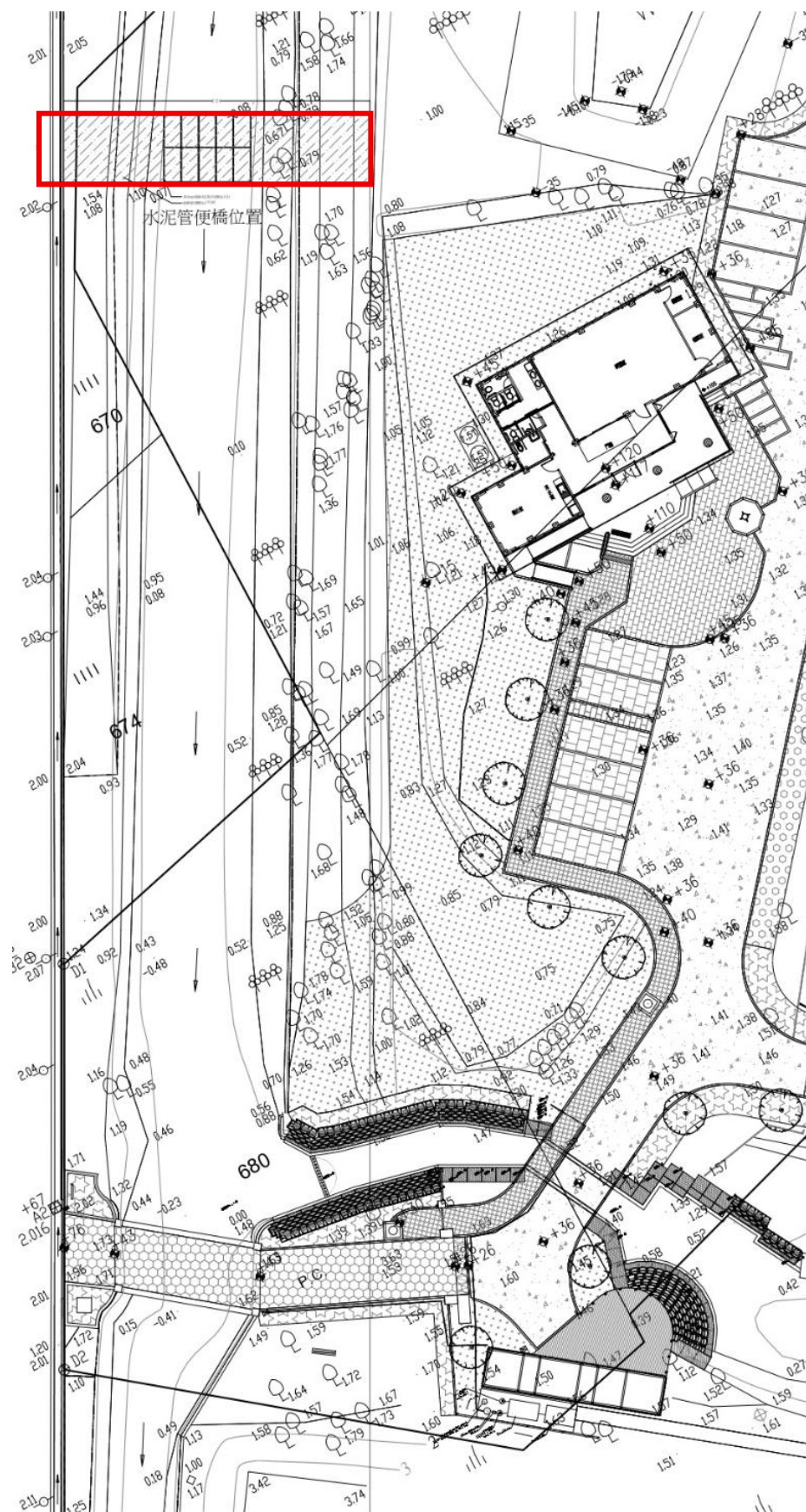
圖 8-8、RC 涵管便道平面位置圖(林愷歆建築師事務所提供)
