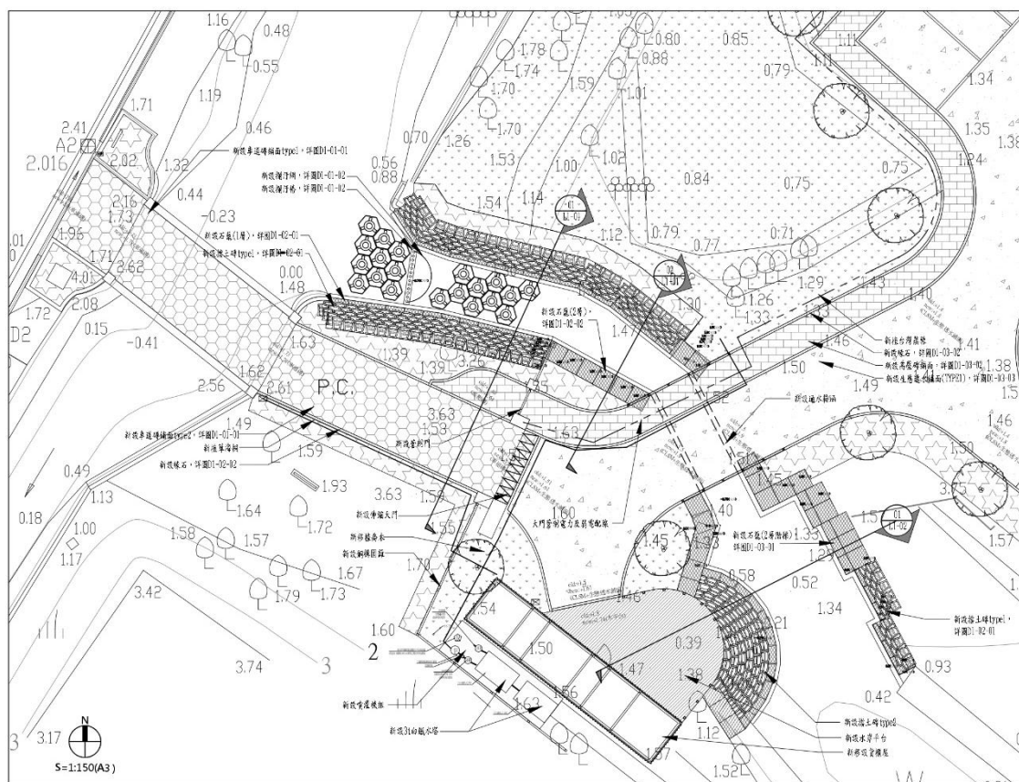
圖 8-2、二期工程補植植栽位置圖(林愷歆建築師事務所提供)
