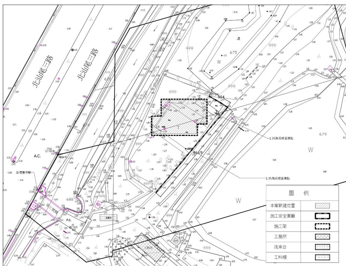
圖 8-10、施工圍籬範圍(林愷歆建築師事務所提供)
