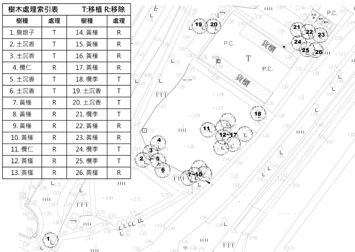
圖 8-1、預計移植及移除樹木位置圖
