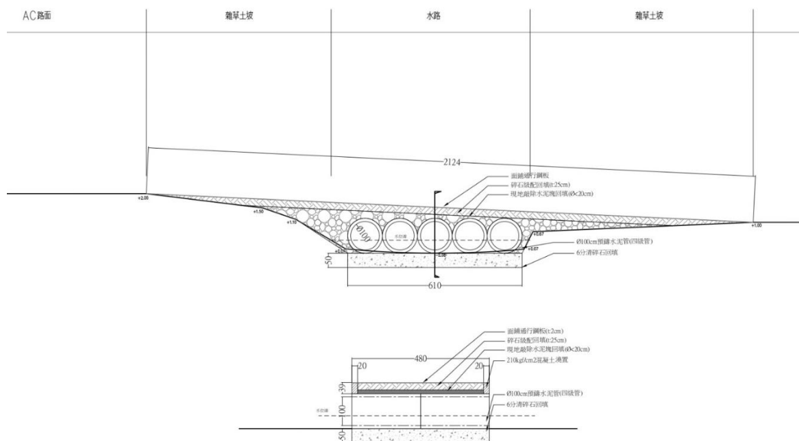
圖 8-7、RC 涵管便道斷面圖(林愷歆建築師事務所提供)
