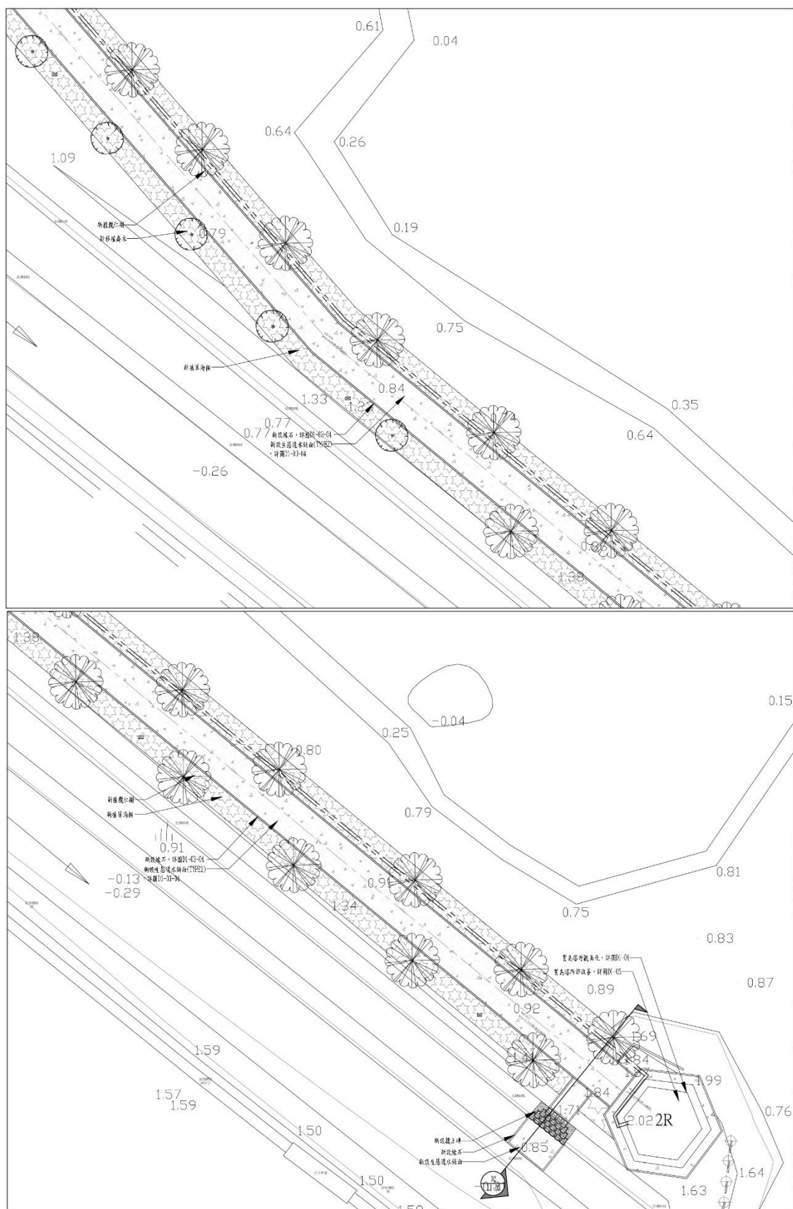
圖 8-3、二期工程(賞鳥步道)植栽分區配置圖(林愷歆建築師事務所提供)
